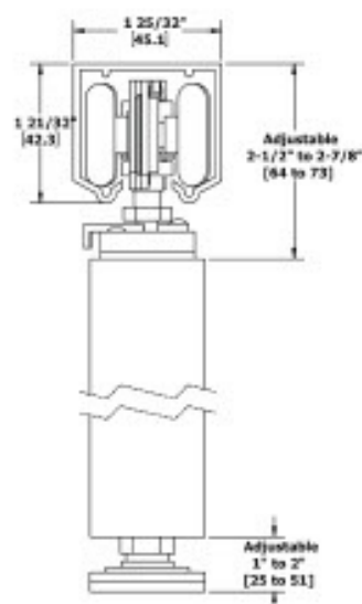
Optional Bottom Track 9121 - 9122
